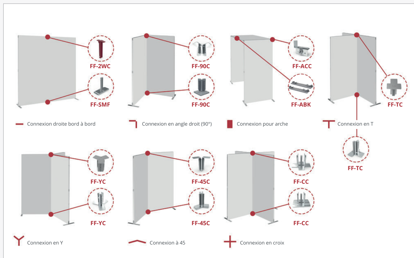
Kit Connecteurs en Y (FF-YC)
